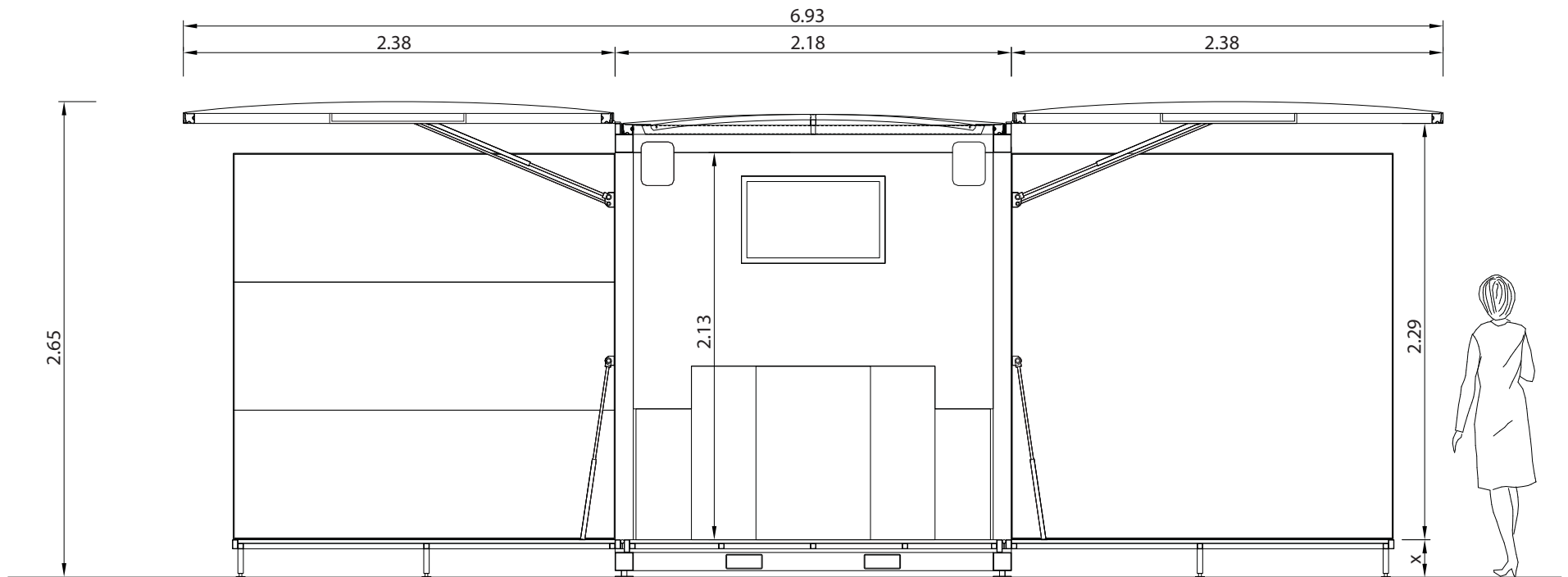
SECCION A-A'
